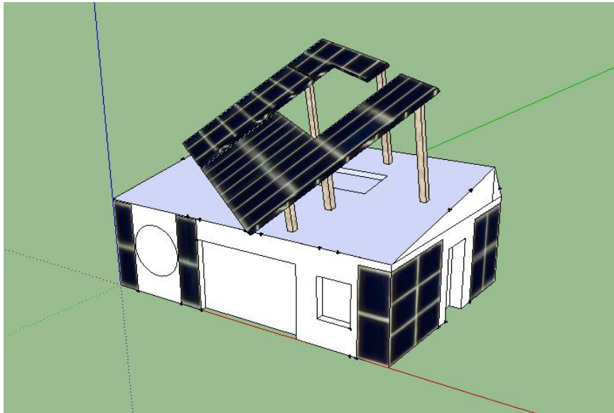
图 6.2-1 最优倾角、朝向示意图
